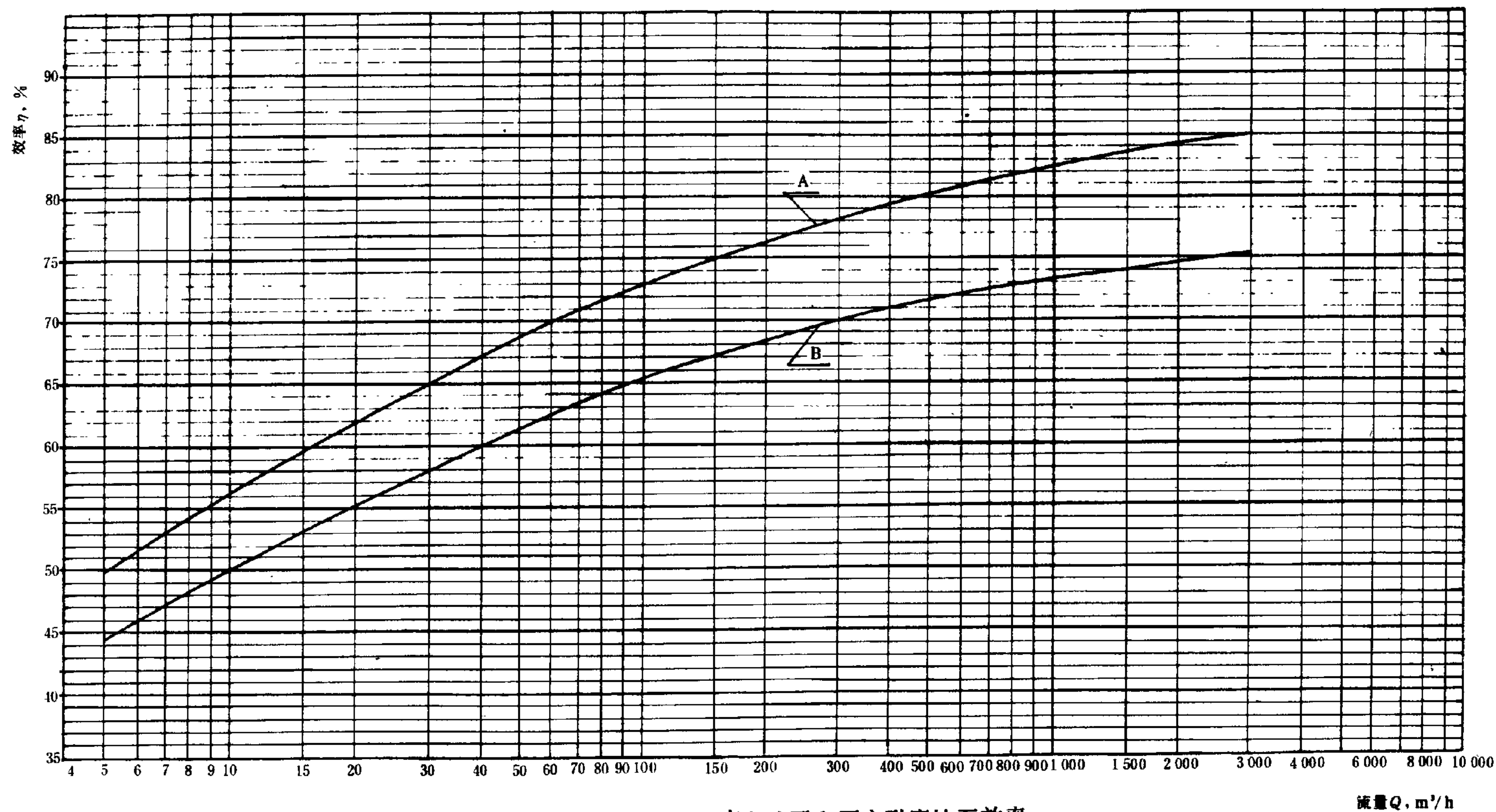
图 3 n_s = 120 \sim 210 离心油泵和离心耐腐蚀泵效率
