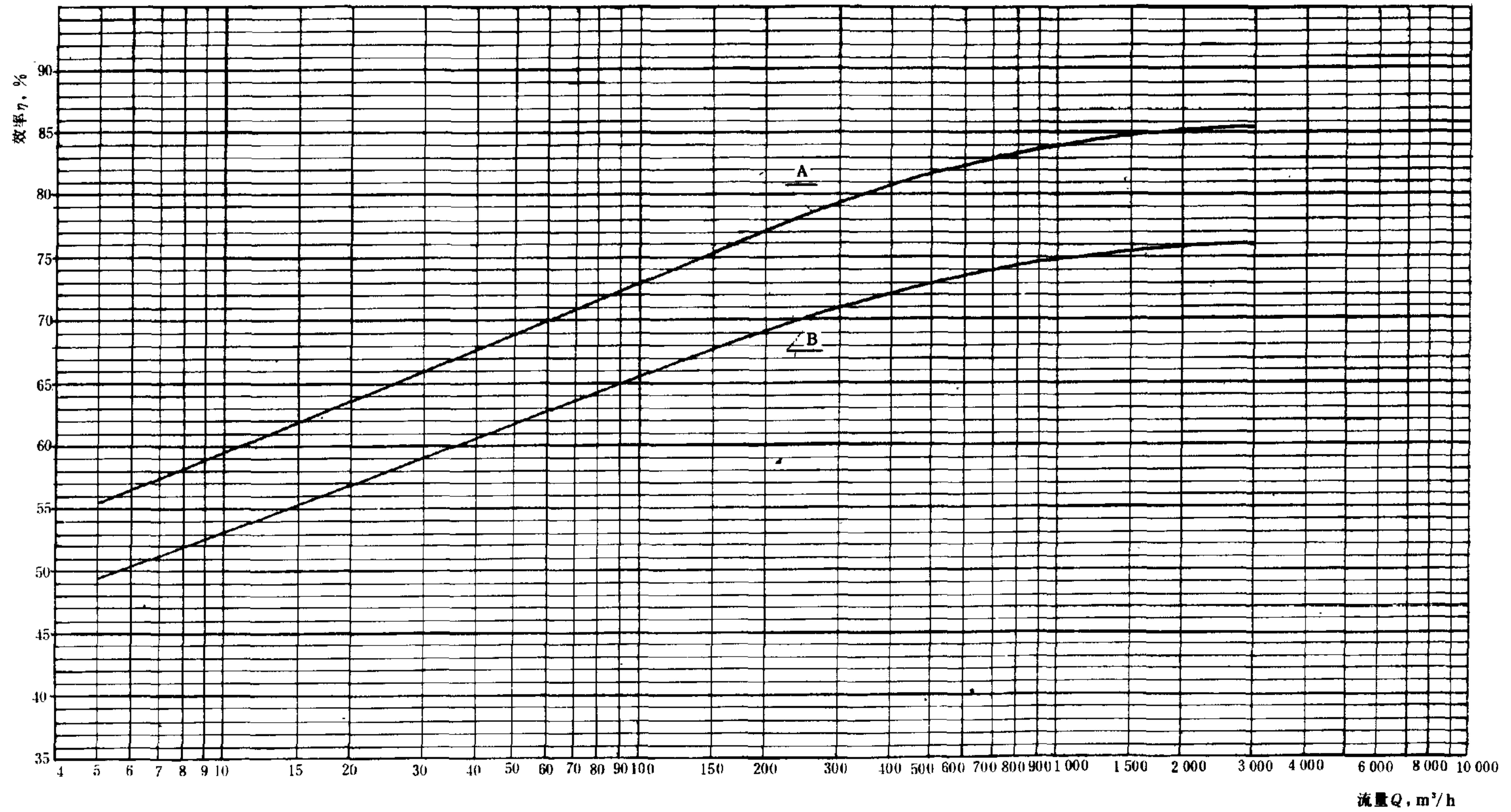
图 2 n_s = 120 \sim 210 多级离心水泵效率
